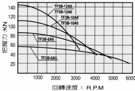
把握力性能曲線 TF3BA
